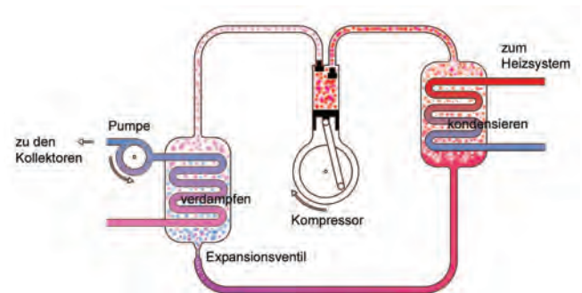
Der Kreislauf einer Wärmepumpe
