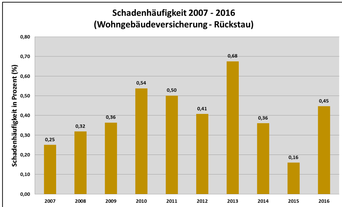
Abbildung 17: Schadenhäufigkeit Rückstau 2007 – 2016; Daten: VHV; Grafik: IFB
